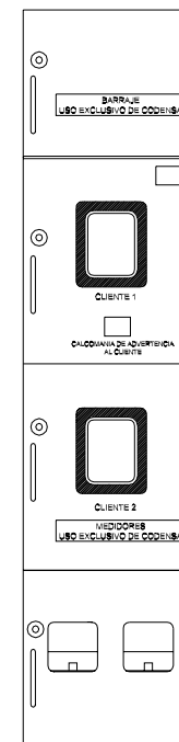
Dos cuentas vertical AE 304-3 ET 905-3
