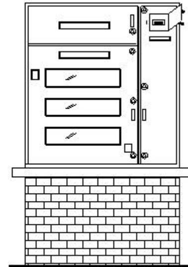
Alternativa Totalizador y barraje lateral
